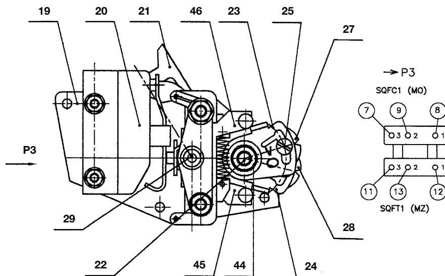
Рис. 2 – Моментный блок
