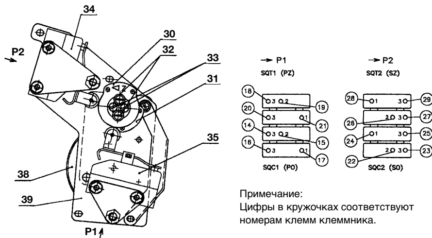
Рис. 3 – Блок положения и сигнализации
