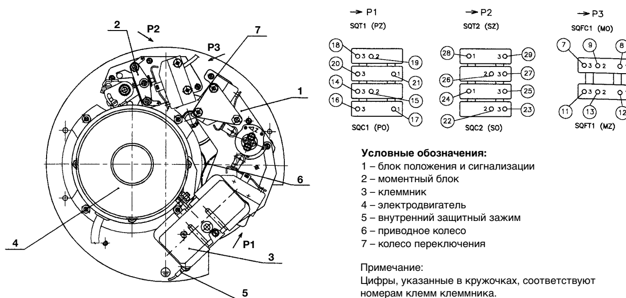
Рис. 1 – Плата управления
