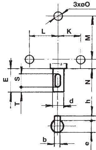
Основная плата - отверстия
