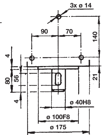
Основная плата - отверстия
