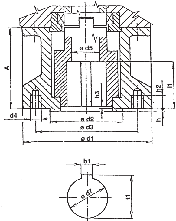
Форма В1 По ČSN EN ISO 5210 (13 3090)
